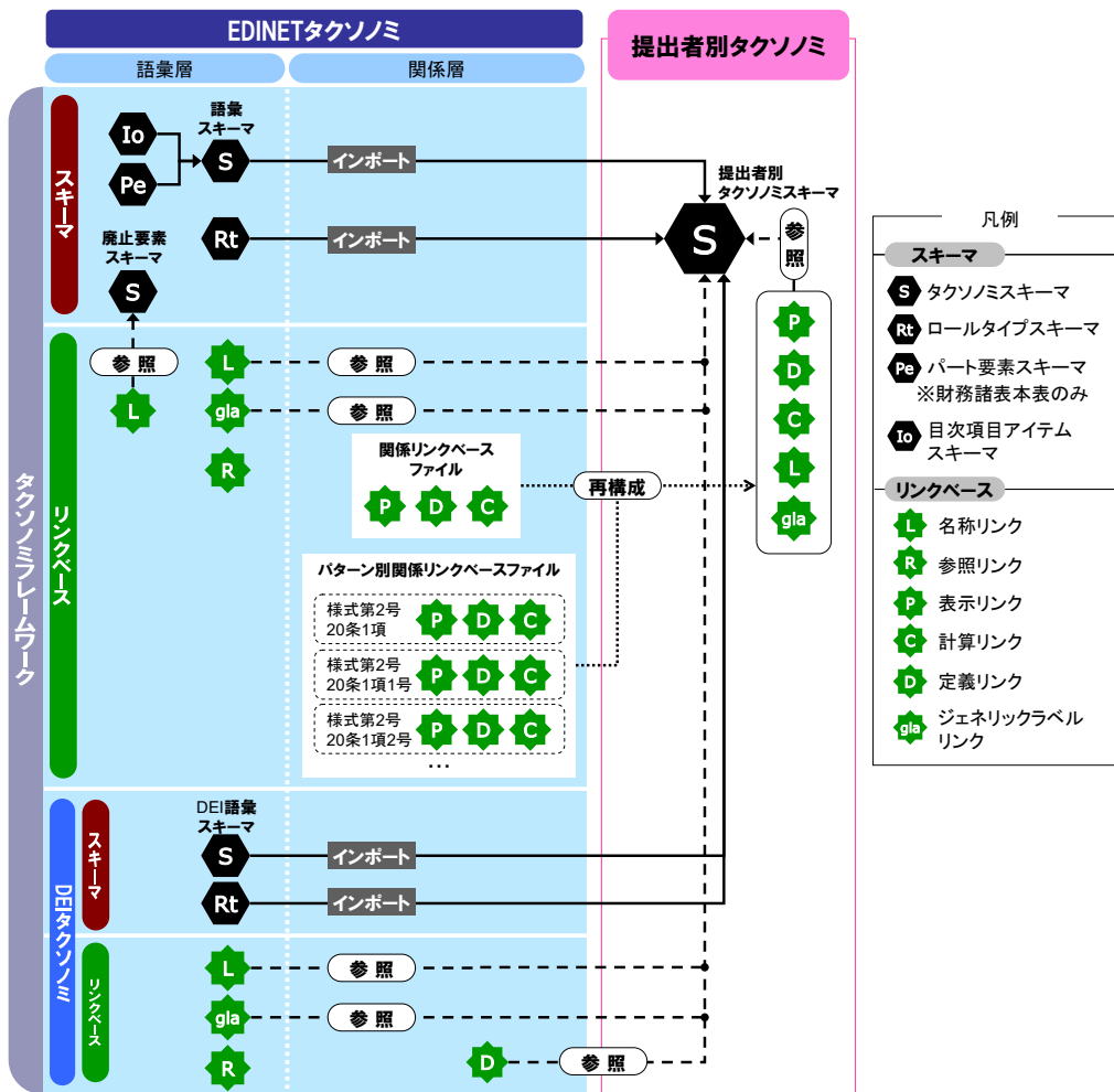
図表 2-1-1 EDINET タクソミの階層
