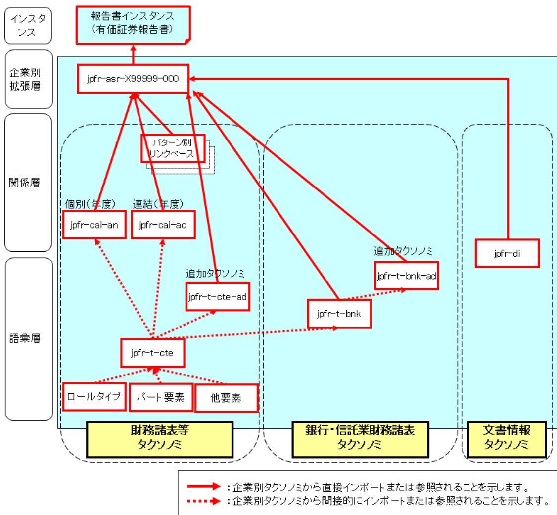
図 3-1 追加タクソミを利用する場合のDTSのイメージ
