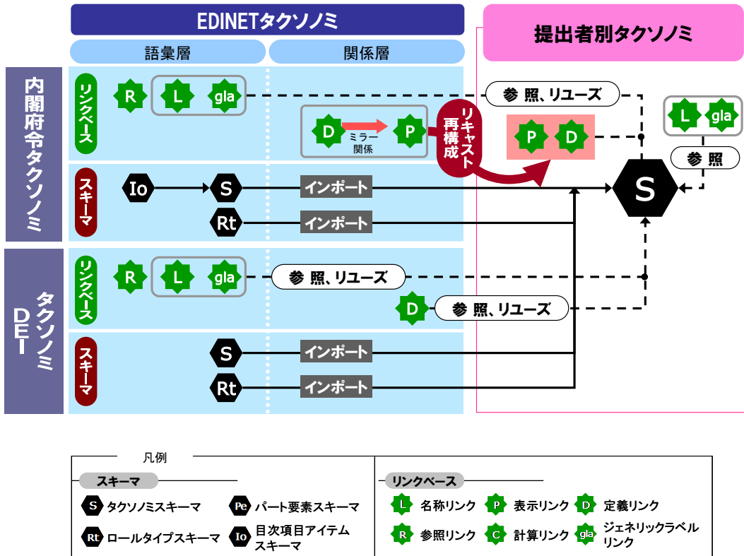
図表 3-2-4 XBRL 対象範囲のパターン(2)
