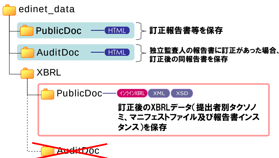
図表 2-1-8 訂正報告書等を提出する場合のフォルダ構成(2)
