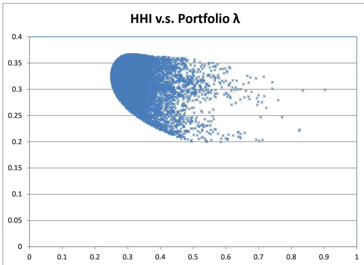
図 7 (d) \rho = 0.8 Dのみ \rho = -0.8
