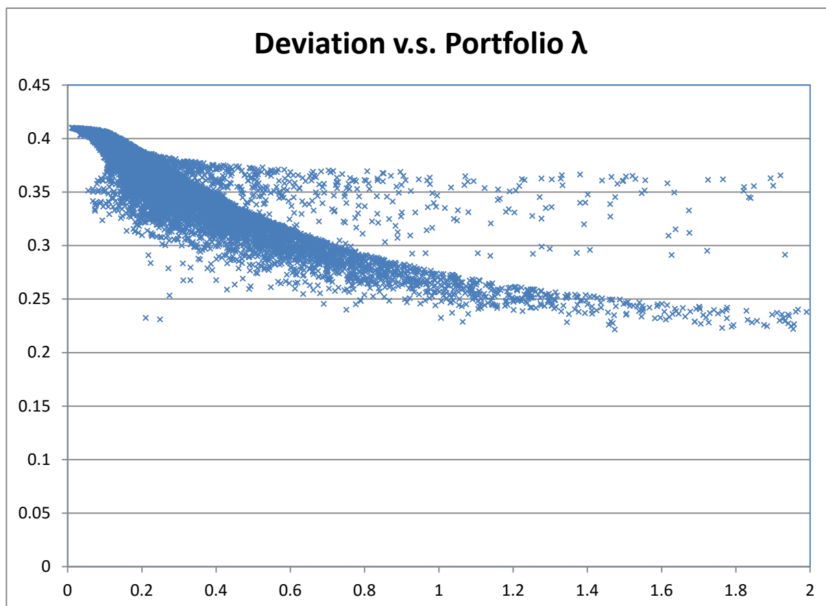
図 11 (d) \rho = 0.8 Dのみ \rho = -0.8
