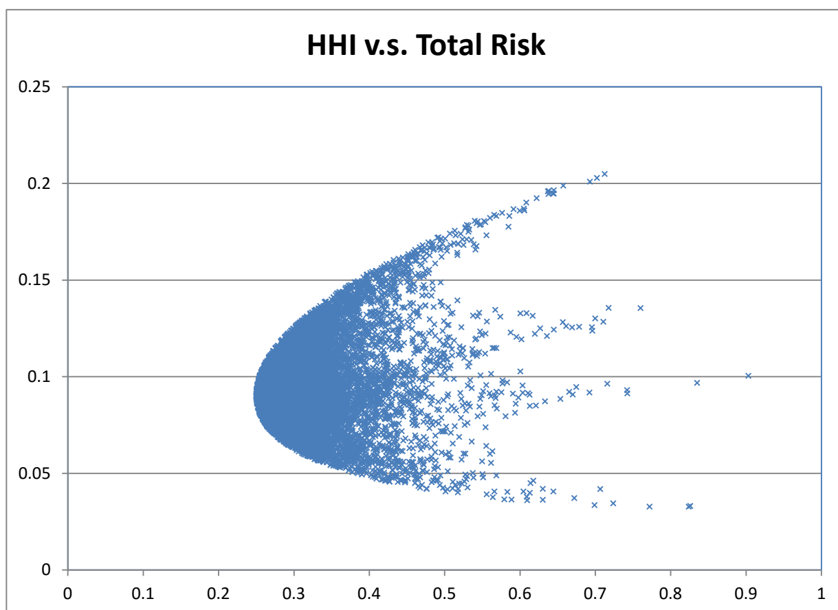
図 8 (d) \rho = 0.8 Dのみ \rho = -0.8
