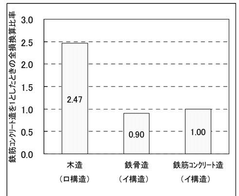
図5-2 2004年新潟県中越地震の被害調査結果比較(日本建築学会「2004年10月23日新潟県中越地震災害調査報告」)
