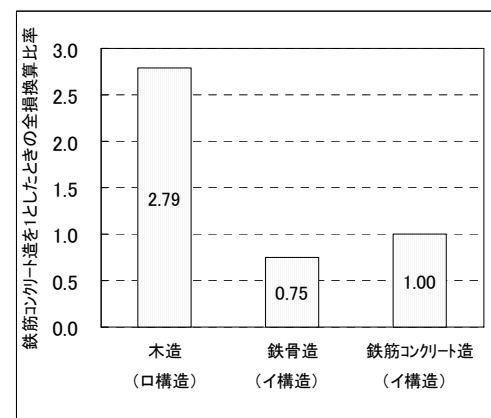
図5-3 2005年福岡県西方沖地震の被害調査結果比較
