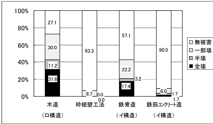
図5-1 1995年兵庫県南部地震の被害調査結果比較(日本建築学会近畿支部「1995年兵庫県南部地震—木造建物の被害—」)
