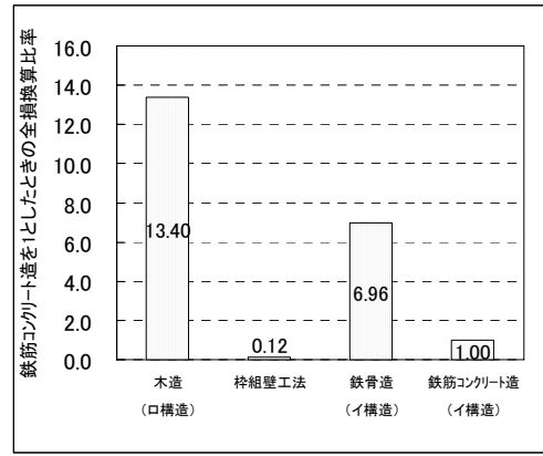
図5-1 1995年兵庫県南部地震の被害調査結果比較(日本建築学会近畿支部「1995年兵庫県南部地震—木造建物の被害—」)
