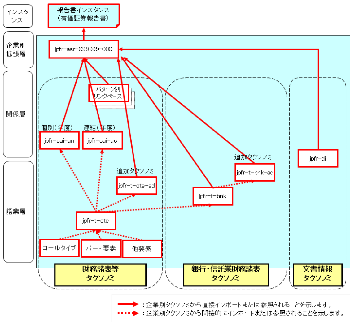
図 3-1 追加タクソノミを利用する場合の DTS のイメージ
