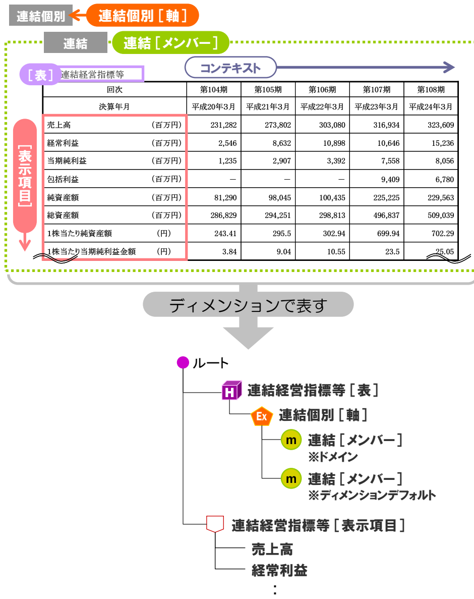
図表 1-5-6 ディメンションで定義される構造のイメージ(連結の場合)
